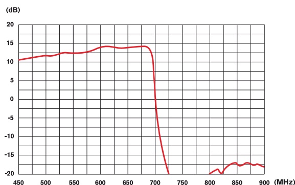
Curva de ganho HyDra 35G
